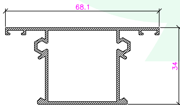
CE-013-0009 Travessa
