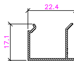
CE-013-0013 Bite
