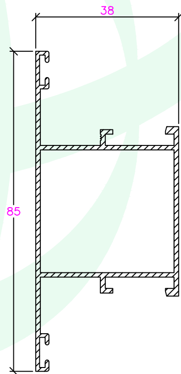
CE-001-38445 Travessa
