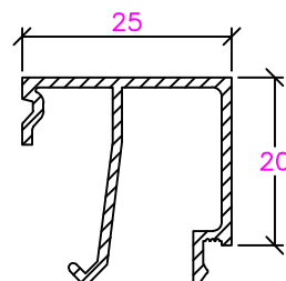
CE-001-38525 Bite
