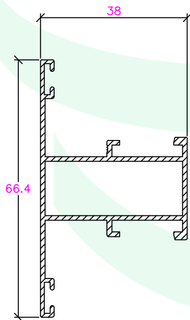
CE-001-38430 Travessa
