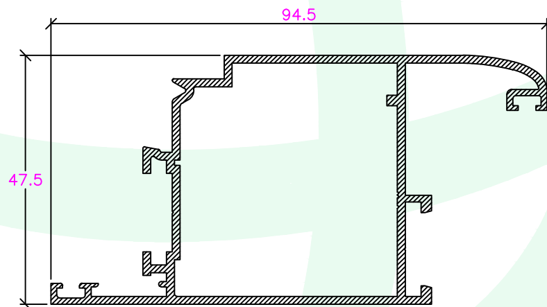
CI-033-40240 Aro Móvel Porta
