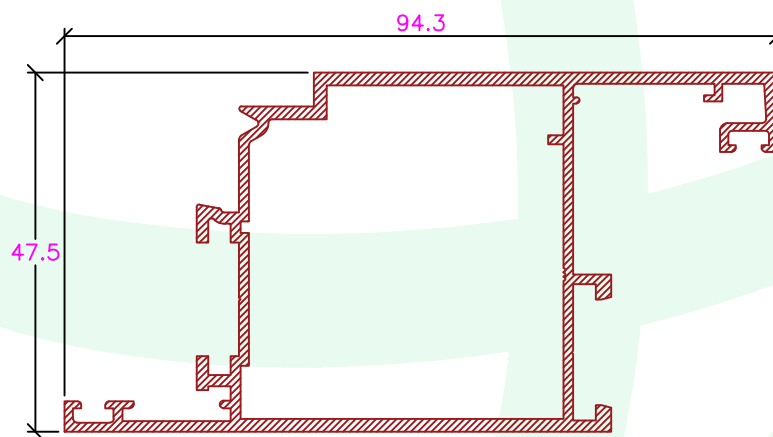
CE-001- 40205 Aro Móvel Porta
