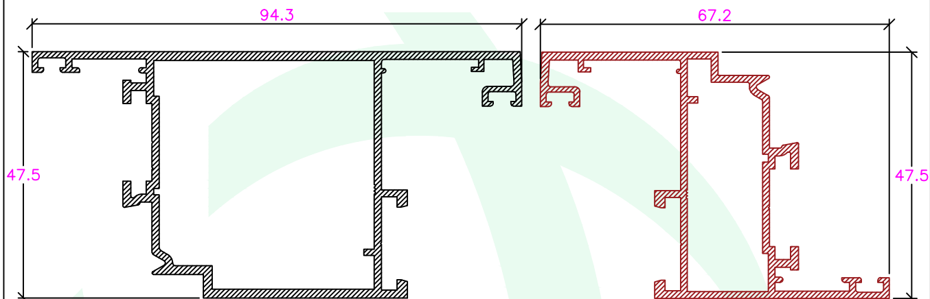
CE-001- 40238 Aro Móvel Porta/Exterior
