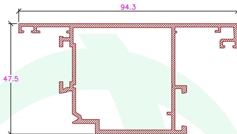
CE-001- 40238 Aro Móvel Porta/Exterior
