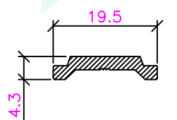
CE-001-40004 Barra Cremone
