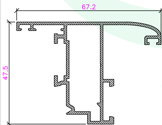
CI-033-40236 Aro Móvel Porta/Exterior
