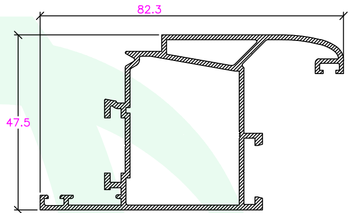
CE-001-40260 Aro Móvel Porta
