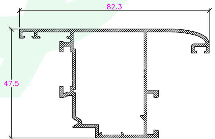
CE-001-40230 Aro Móvel Porta/Exterior
