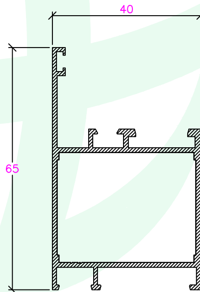
CI-033-40140 Aro Fixo
