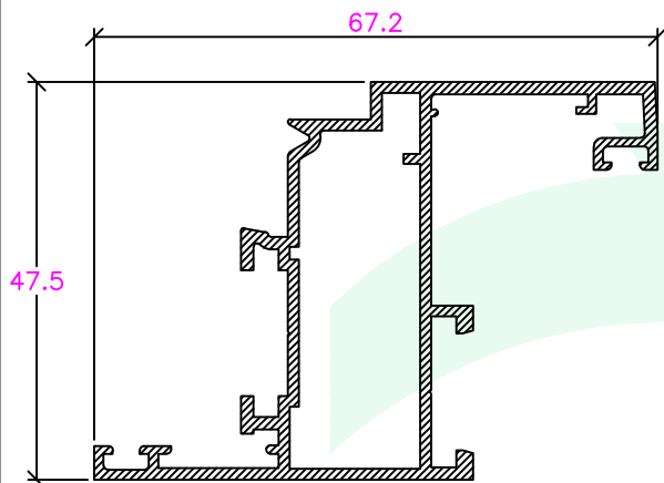
CE-001- 40200 Aro Móvel Janela
