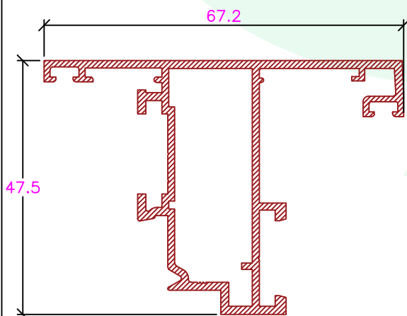
CE-001-40237 Aro Móvel Porta/Exterior
