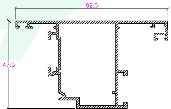
CE-001- 40232 Aro Móvel Porta/Exterior
