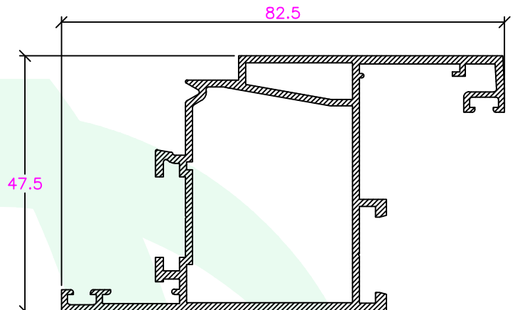
CE-001-40250 Aro Móvel Porta
