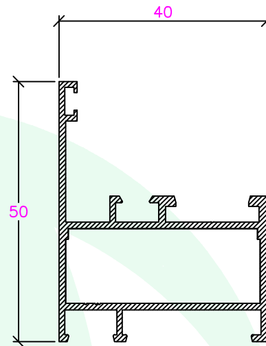
CI-033-40100 Aro Fixo
