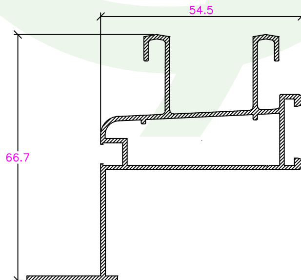
CE-001-61100 Aro fixo Apainelado
