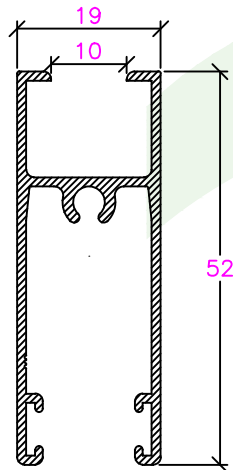
CE-001-61022 Aro Móvel Horizontal
