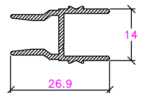
CE-001-61018 Perfil 3 / 4 Folhas
