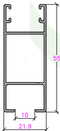
CE-001-61025 Aro Móvel Lateral
