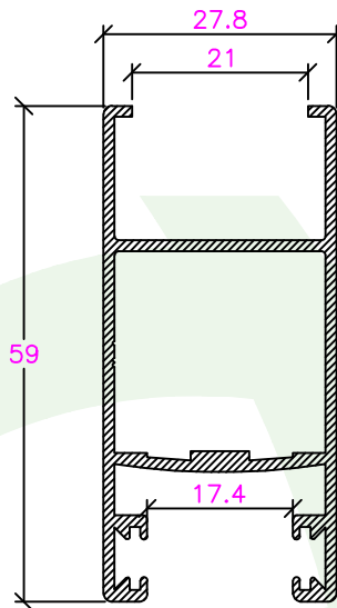
CI-057-0037 Aro Móvel Lateral Vidro Duplo
