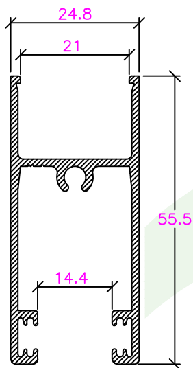
CI-057-0041 Aro Móvel Horizontal Vidro Duplo
