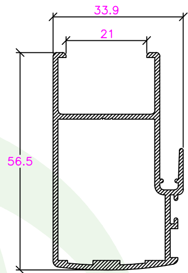
CI-057-0040 Aro Móvel Central Vidro Duplo
