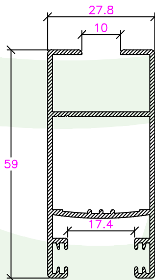
CI-004-0059 Aro Móvel Lateral Vidro Simples
