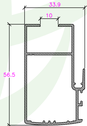
CI-004-0060 Aro Móvel Central Vidro Simples
