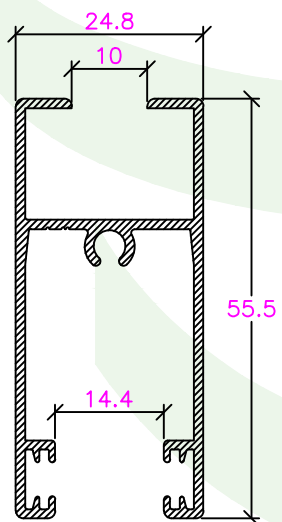
CI-004-0061 Aro Móvel Horizontal Vidro Simples
