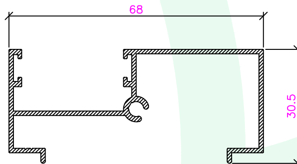
CE-013-0003 Ombreira
