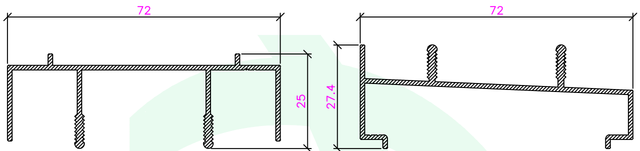
CE-013-0001 Padieira
