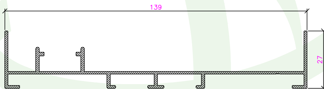
CE-001-90028 Ombreira Tri-Rail
