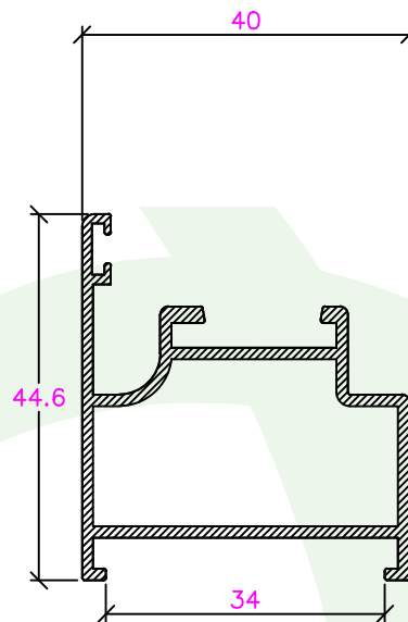
CI-004-0040 Aro Fixo
