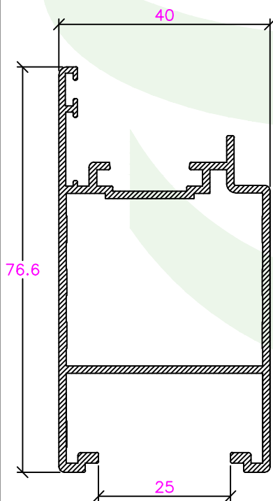
CI-004-0042 Aro Fixo/Móvel Largo
