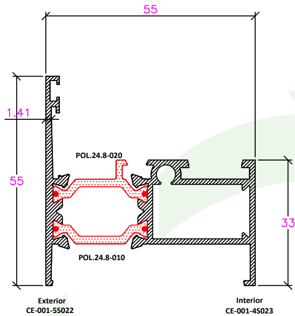
Aro Fixo CI-033-55105
