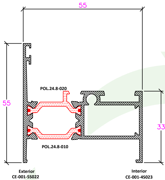
Aro Fixo CI-033-55105
