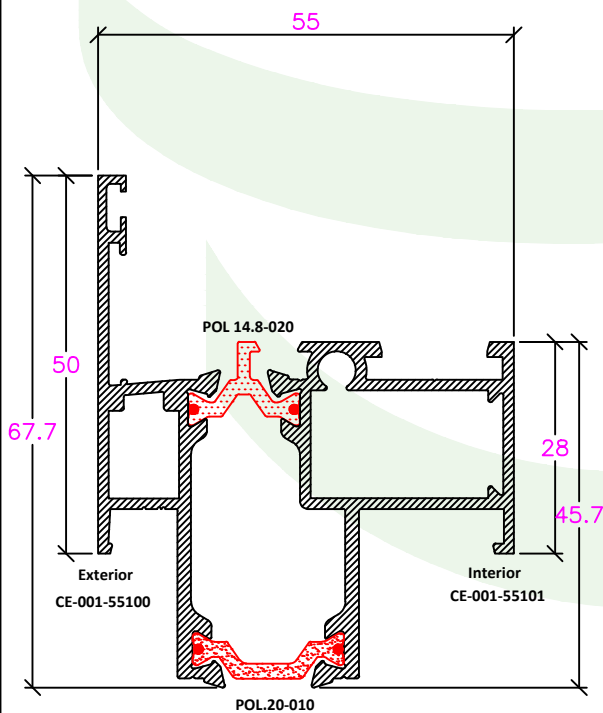
Aro Fixo/Lig. Fachada CI-033-55115
